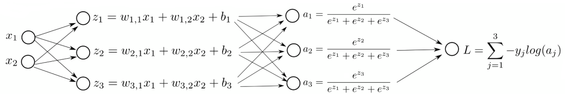
Figura 4.2: Flusso della regressione softmax con due ingressi e tre classi: dai logiti z_i = w_{i,1}x_1 + w_{i,2}x_2 + b_i alle probabilità a_i = \frac{e^{z_i}}{\sum_{k=1}^3 e^{z_k}} , fino alla loss a entropia incrociata L = \sum_{j=1}^3 -y_j \log(a_j) .
